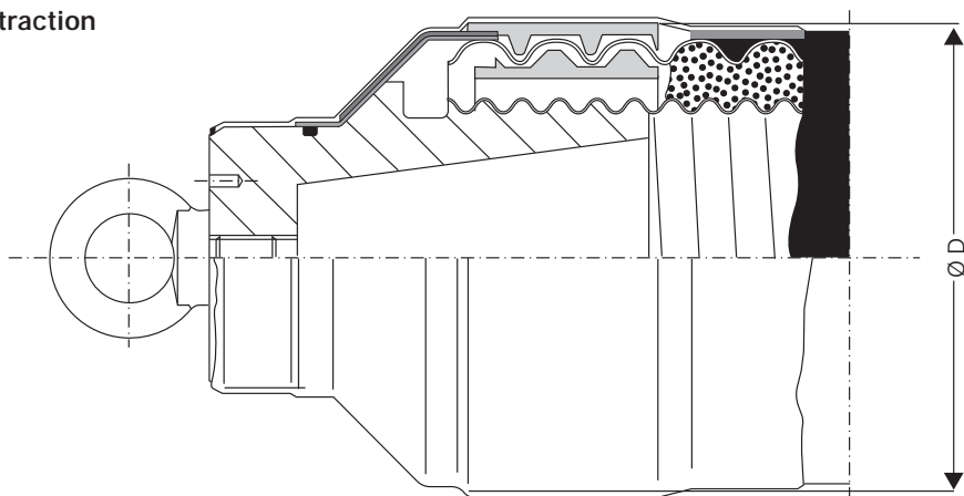
Tête de traction
