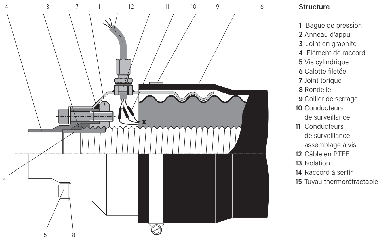
Figure 1: Raccord avec joint circulaire en graphite de type GR
