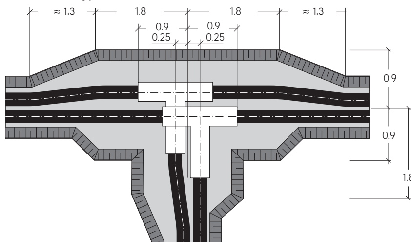
Figure 1: Raccordement, espace de travail (vue d'en haut) Les cotes indiquées s'appliquent à tous les types FHK
