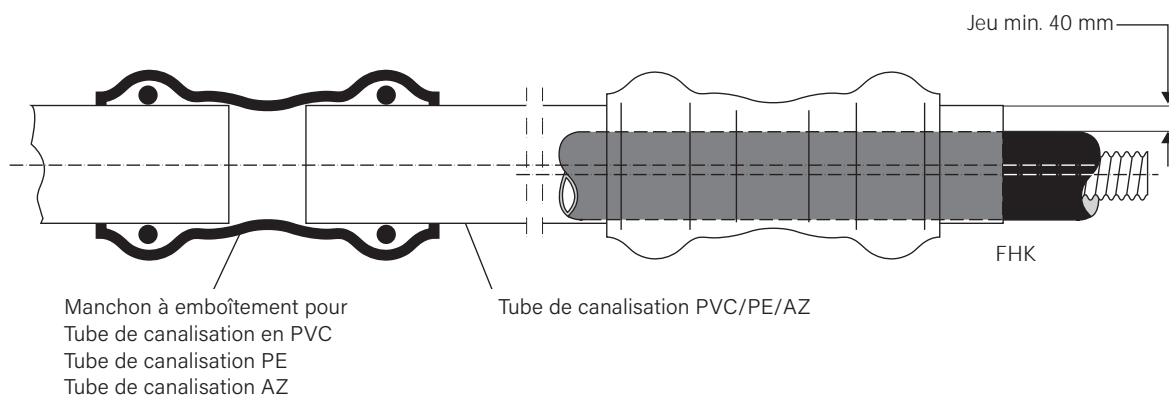
Figure 1: Pose FHK avec des tubes protecteurs droits sans déports, avec patins de glissement. Longueur du tube protecteur ≥ 50 m uniquement après consultation avec BRUGG
