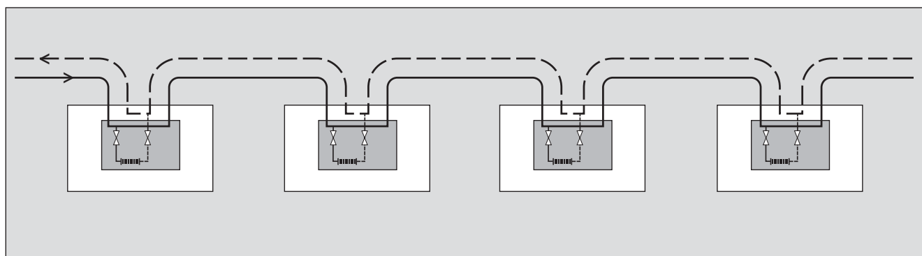
Fig. 2 Méthode de bouclage, raccords dans les bâtiments
