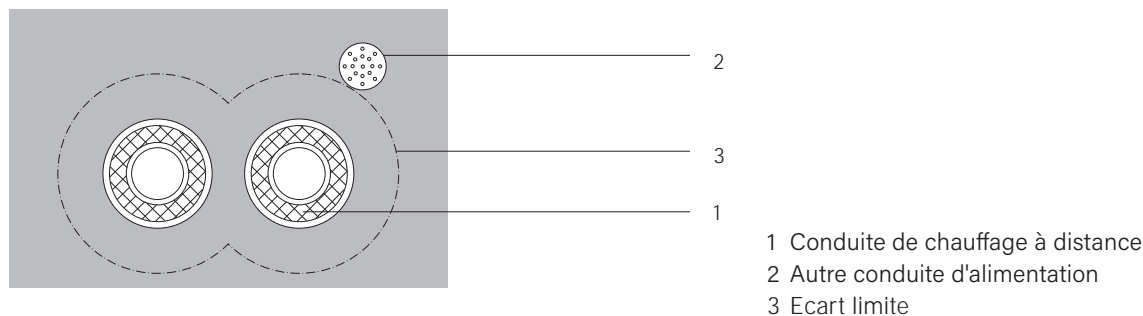
Figure 1: Conduites posées en parallèle
