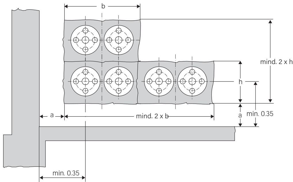
Figure 4: Ouverture de mur avec la méthode de bouclage
