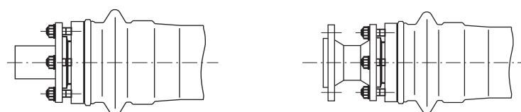
Figure 2: Types d'exécution du raccord
