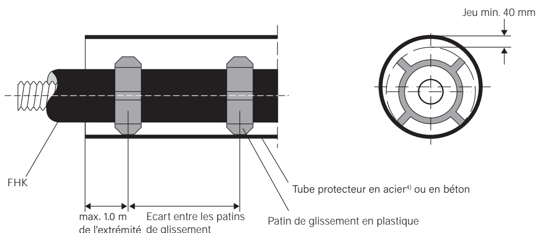
Figure 1: Pose FHK avec des tubes protecteurs droits sans déports, avec patins de glissement. Longueur du tube protecteur ≥ 50 m uniquement après consultation avec BRUGG
