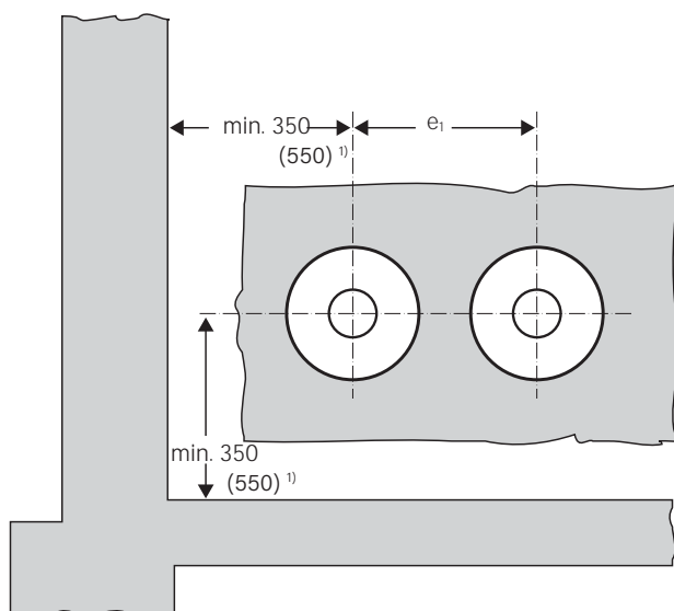
Figure 2: entraxe et écartement du mur
