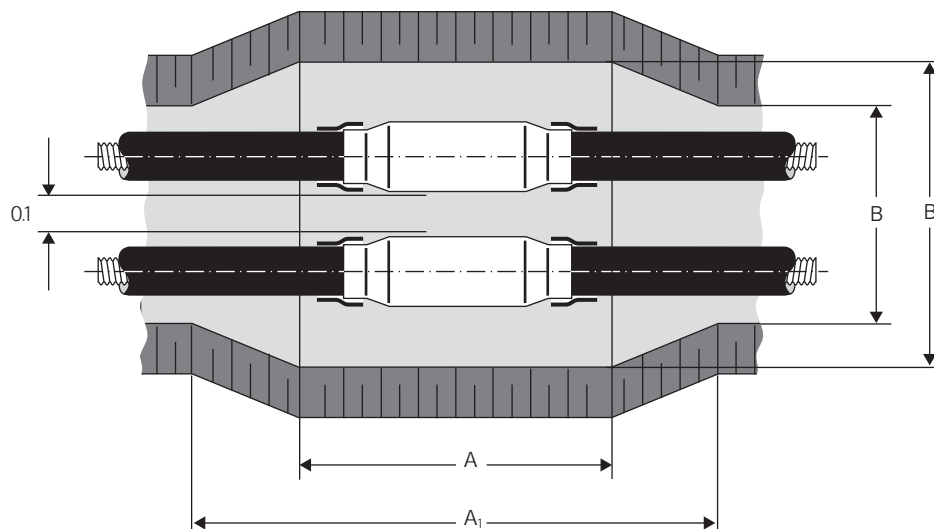
Figure 2: Espace de travail pour le raccord de couplage (vue de dessus)
