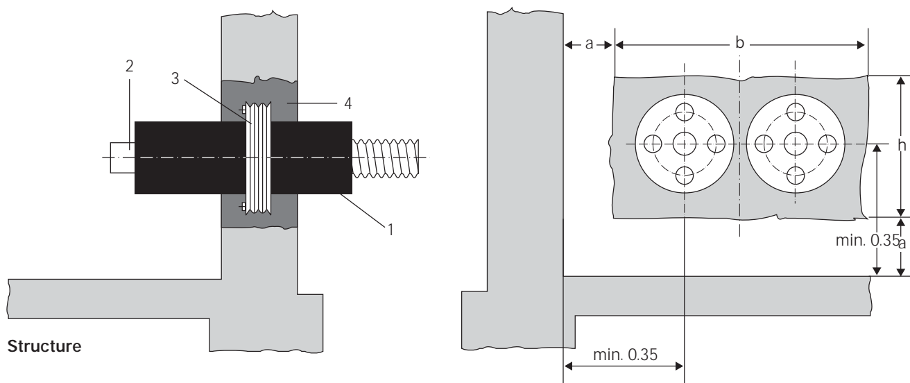
Figure 3: Ouverture de mur pour le raccord FLEXWELL
