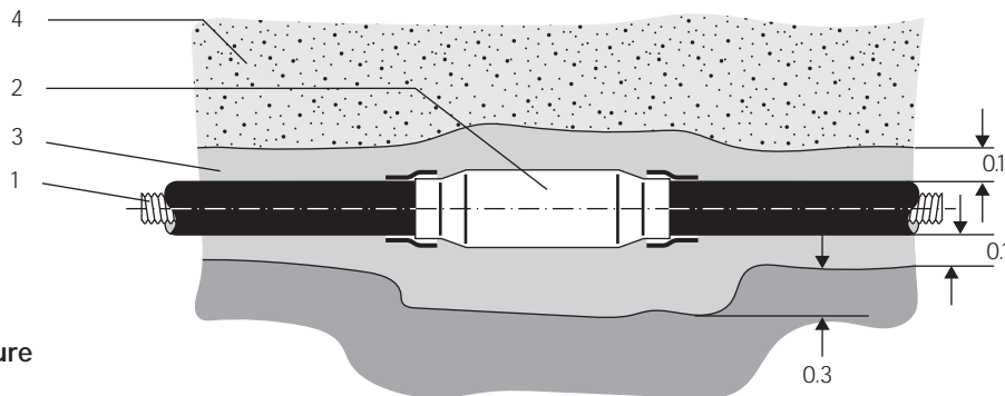
Figure 1: Espace de travail pour le raccord de couplage (vue latérale)
