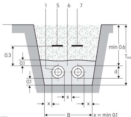
Figure 2: coupe de la fouille Coupe A-A
