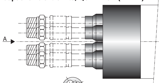
Capuchon d'extrémité, QUADRIGA (PE-LD)
