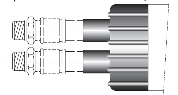
Capuchon d'extrémité thermorétractable, QUADRIGA
