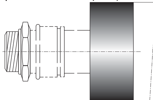
Capuchon d'extrémité, DUO (PE-LD)
