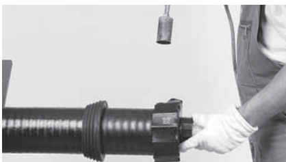
7 Procéder à la rétraction du capuchon d'extrémité CPX pour locaux humides, selon les instructions de montage Raychem-DHEC, ou monter le capuchon d'extrémité CPX pour locaux secs.
