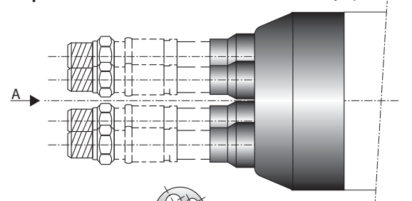
Capuchon d'extrémité thermorétractable, QUADRIGA
